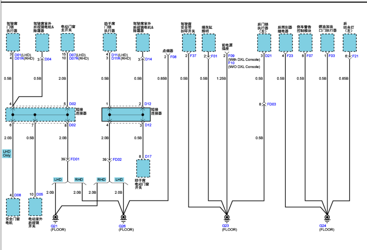
搭铁分布(6)
